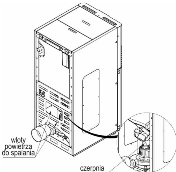
Rysunek 11. Czerpnia powietrza - otwór dolotowy powietrza.
