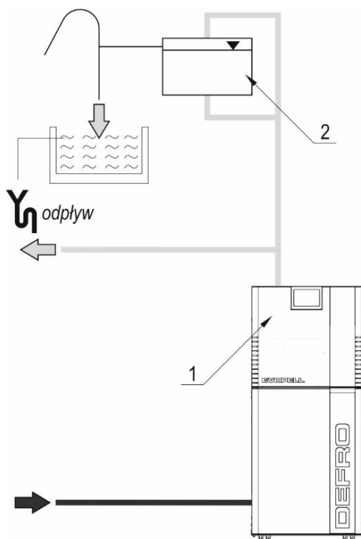
Rysunek 5. Przykładowy schemat zabezpieczeń kotła EVOPELL w układzie otwartym
