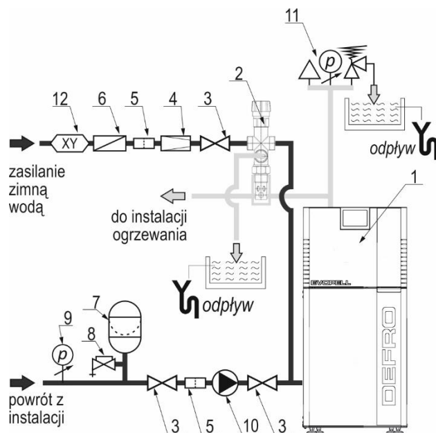
Rysunek 6. Przykładowy schemat zabezpieczeń kotła w układzie zamkniętym:
